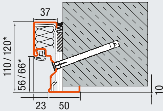
DryFix Zarge mit Diagonalbefestigung (Sichtmauerwerk / Beton)
